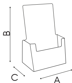
PDB102 DIMENSIONE INTERNA SCOMPARTI Larghezza: 110 mm Profondità: 32 mm
